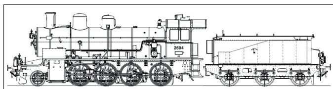
SBB C 4/5 2604
